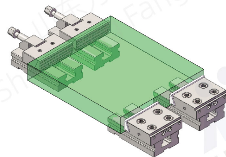
动钳组件与定钳组件配合使用, 将工件压紧于钳体面上
