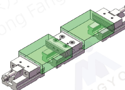
动钳口组件与双向定钳口组件配合使用
