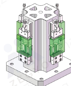
定动钳组件与方箱配合使用。
